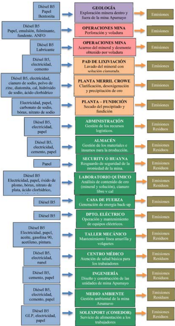
Figura 4. Ingresos y salidas en mina Apumayo (Solórzano, 2019). Figure 4. Inputs and outputs diagram of Apumayo mine (Solórzano, 2019).
