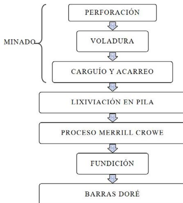
Figura 1. Etapas del Proceso de Producción de Oro en la mina Apumayo. (Mina Apumayo, 2018).
