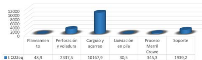
Figura 6. Emisiones de alcance 1 por proceso de la mina Apumayo (Solórzano, 2019).
