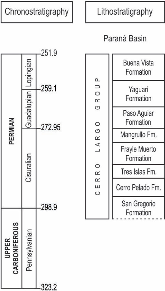
Figure 3. Pennsylvanian-Permian lithostratigraphic units of the Paraná Basin in Uruguay (based on de Santa Ana et al. , 2006; Beri et al. , 2011). Figura 3. Unidades litoestratigráficas de edad Pennsylvaniano-Pérmico correspondientes a la Cuenca Paraná en Uruguay (basado en de Santa Ana et al. , 2006; Beri et al. , 2011).
