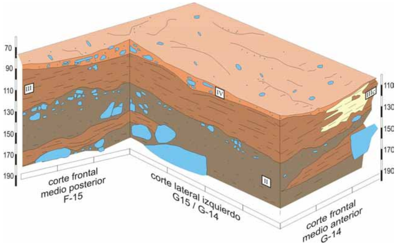
Figura 9. Secciones litoestratigráficas en el corte 7 (2014) (cuadrículas F-G/13-14-15).
