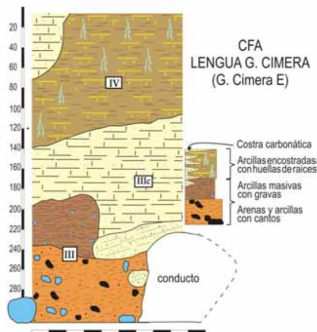
Figura 14. Secciones litoestratigráficas en Trinchera Salomón (2012) y en Lengua - Galería Címera / Salomón (2013).
