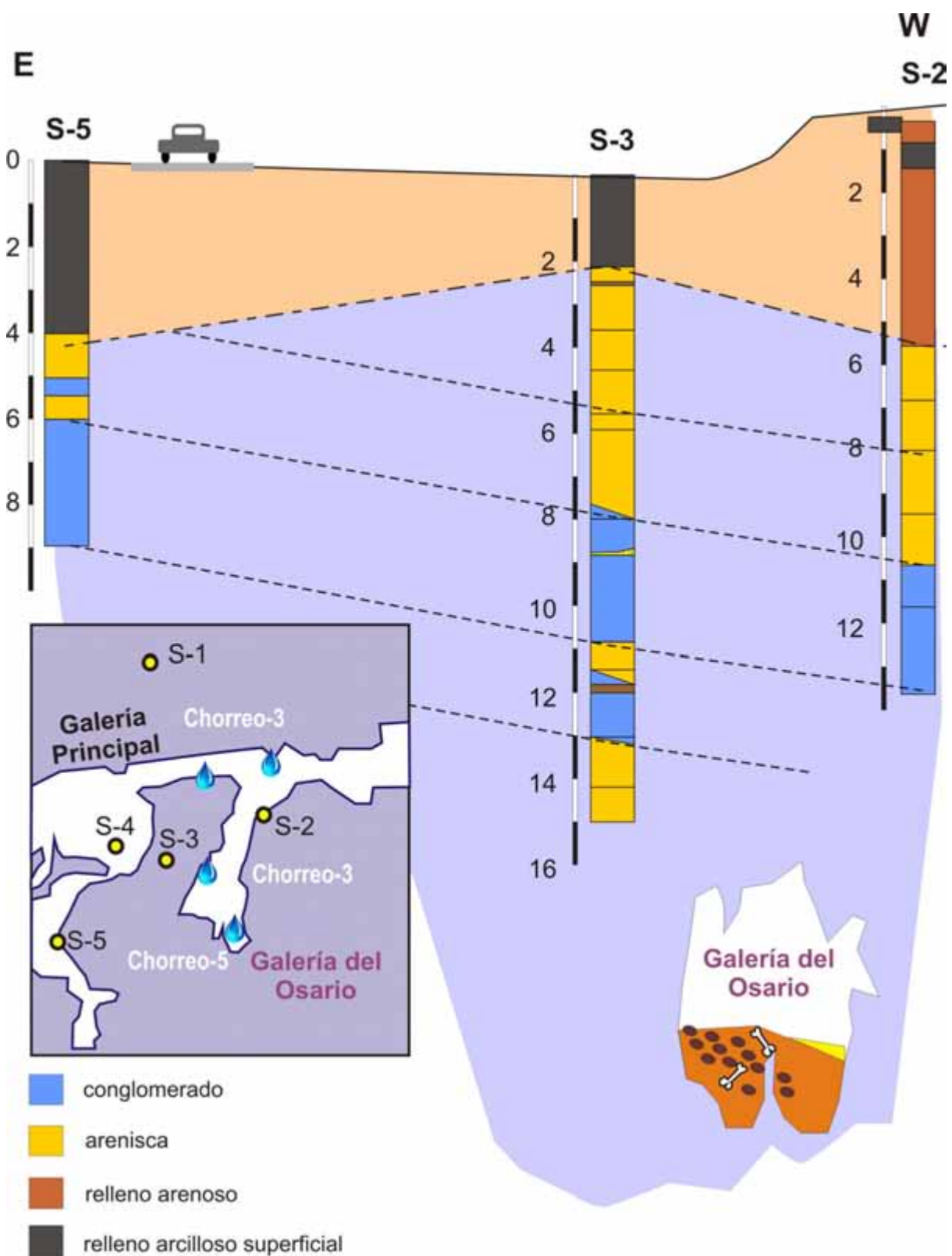
Figura 2. Correlación de los sondeos S-2, S-3 y S-5 en un perfil E-O, indicando la posición relativa de la zona de la Galería del Osario. Se indica dónde percolaron ("chorreos") los lodos de sondeo en el interior de la cueva durante las labores en 2006.
