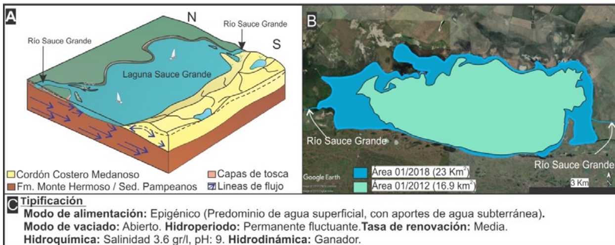
Figura 3. A) Modelo de hidrogeológico de la Laguna Sauce Grande. B) Variaciones areales de la laguna. C) Tipificación hidrológica.
