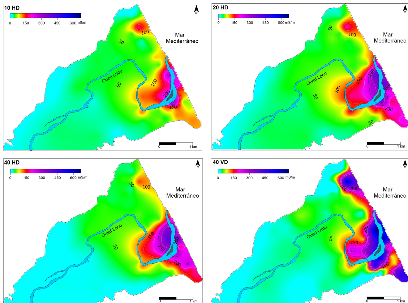
Figura 6. Mapas de conductividad aparente obtenida a partir de las configuraciones entre bobinas 10 HD, 20 HD, 40 HD y 40 VD. Figure 6. Electrical resistivity cross-sections from different configuration between coils of 10 HD, 20 HD and 40 VD.
