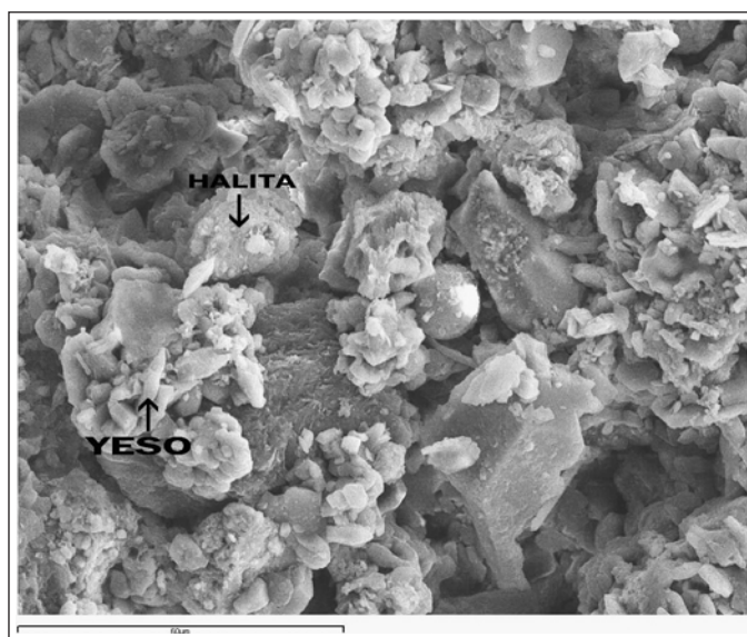
Figura 14. Parte externa de una muestra de arenisca del monumento observada y analizada al SEM+EDX, con partículas de contaminación, halita y yeso
