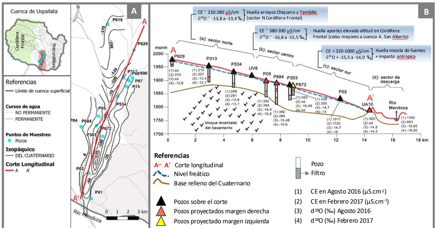
Figura 4. Modelo conceptual preliminar del acuífero del Valle de Uspallata. [A] Mapa isopáquico del relleno cuaternario, posición de los pozos de muestreo y traza de corte longitudinal. [B] Corte longitudinal del valle con posición relativa de los pozos y sus correspondientes valores de conductividad eléctrica (CE) y \delta^{18}O en Agosto 2016 (invierno) y Febrero 2017 (verano).
