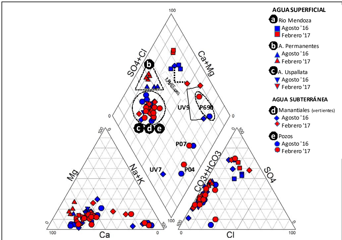
Figura 2. Diagrama de Piper de las muestras de las campañas de agosto 2016 (invierno) y febrero 2017 (verano). Figure 2. Piper diagram showing the samples of August 2016 (winter) and February 2017 (summer) campaigns.
