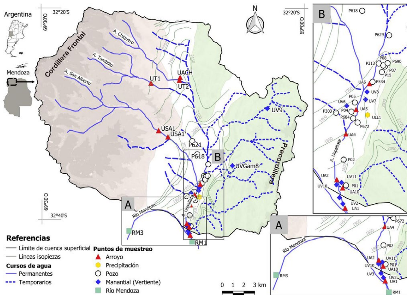
Figura 1. Izquierda: Mapa de la zona de estudio mostrando una piezometría regional tentativa y los sitios de muestreo. [A] Detalle del sector de descarga del A. Uspallata en el río Mendoza. [B] Detalle de la zona central del Valle de Uspallata.
