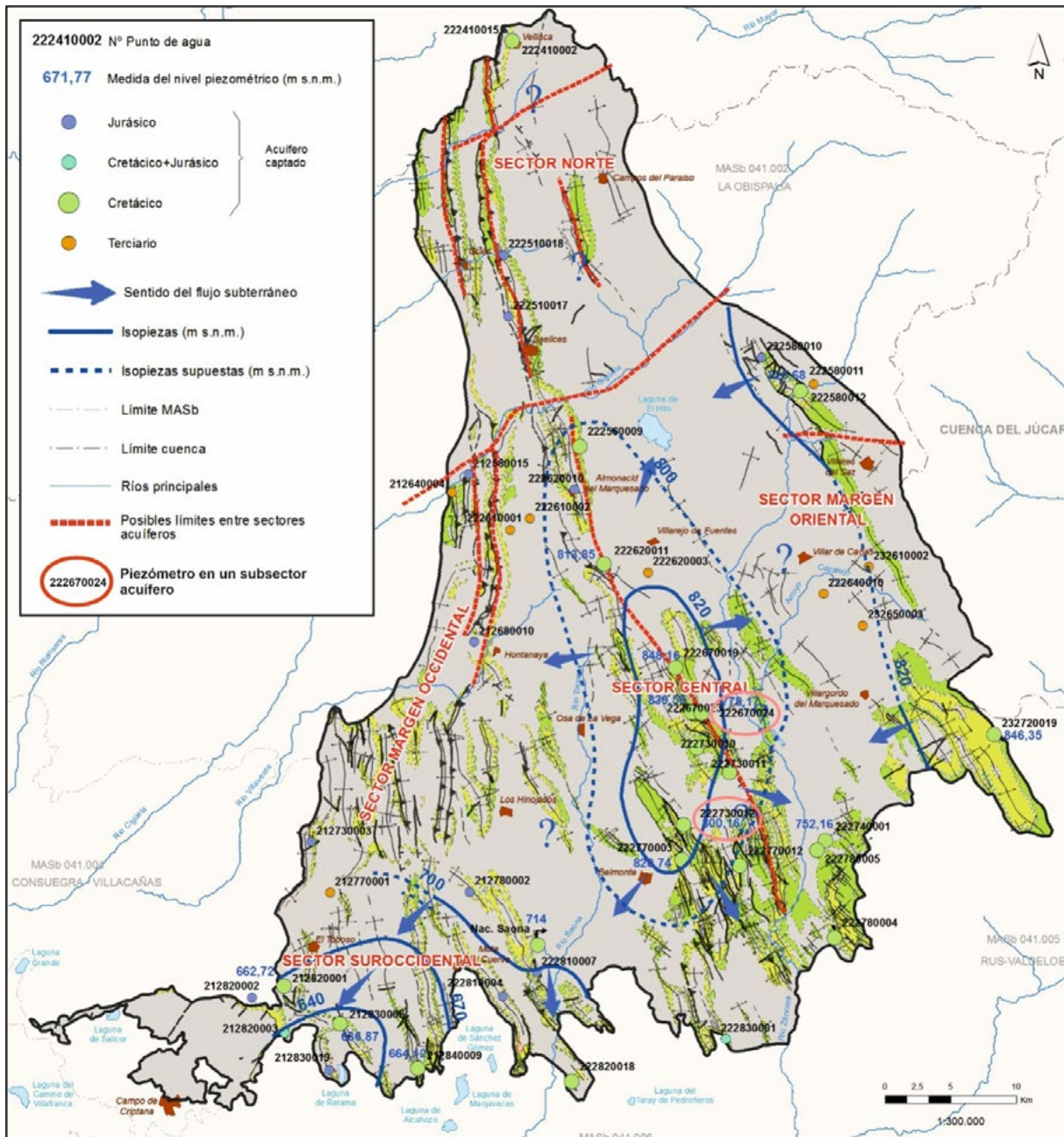
Figura 5. Sectorización del acuífero Cretácico a partir de la piezometría. (datos de octubre de 2018). En Domínguez et al., 2018 a. Figure 5. Sectorization based on the piezometry of the Cretaceous aquifer (data from October 2018). From Domínguez et al., 2018 a.
