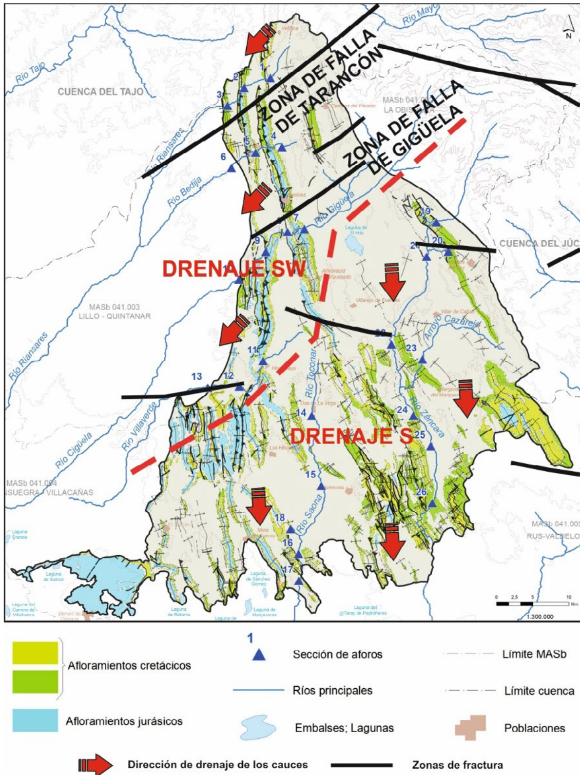
Figura 10. Ríos de la MASb Sierra de Altomira. Secciones de aforo. Principales estructuras transversales y direcciones de drenaje de los cauces. Modificado de Domínguez et al., 2018 b. Figure 10. Rivers in the Sierra de Altomira GWB. Flow measurement sections. Main transverse structures and river drainage direction. Modified from Domínguez et al., 2018 b.
